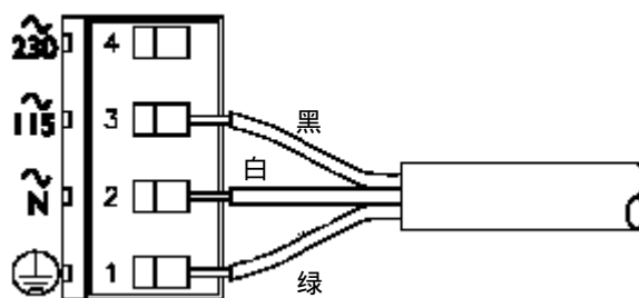
图 2-11 连接 115V 单相电源到 序列号前缀为“A”或无的测定仪
