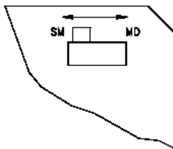
图 3-2 SINGLE MODE/MULTI-DROP(单模式/多点)切换开关的位置（仅针对配有 HART 的测定仪）
