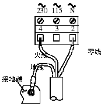
图 2-9 连接 230V 单相电源到序列号前缀为“B”的测定仪
